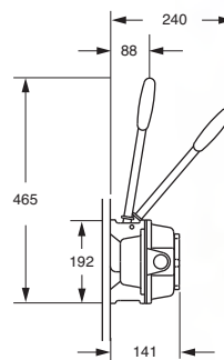
BP 0527 Vista laterale
