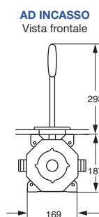
IN COPERTA Vista frontale
