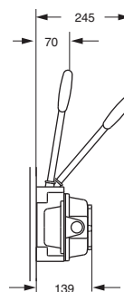
A PARATIA Vista laterale
