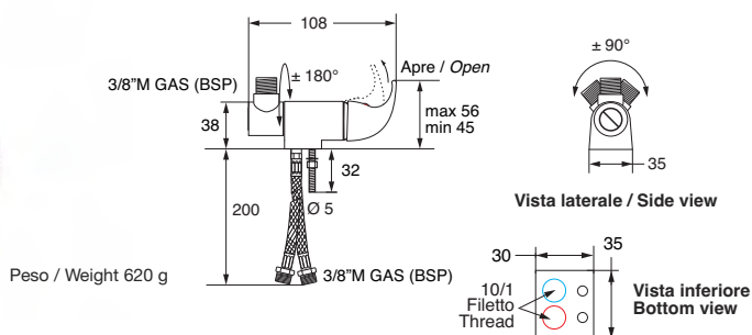
Maniglia / Handle PUFFO 1
