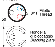
Vista inferiore / Bottom view
