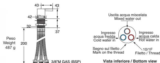
Maniglia / Handle SIMPLY MINI
