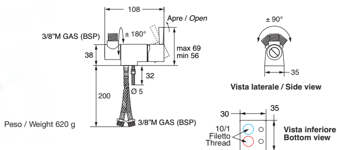
Maniglia / Handle SIMPLY MINI
