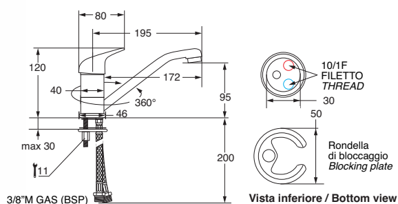
Vista inferiore / Bottom view
