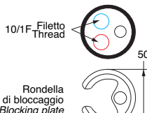
Vista inferiore / Bottom view
