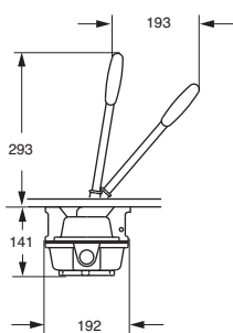
BP 0535 Vista laterale
