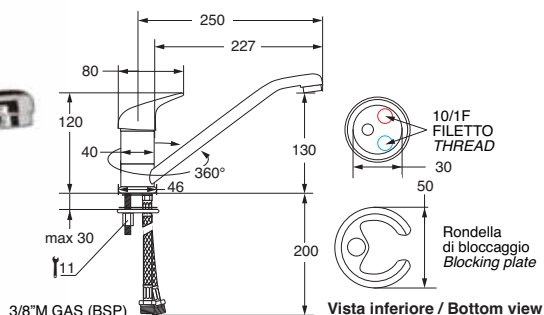
Vista inferiore / Bottom view
