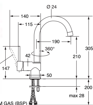
Optional MYL 1501 cod. 03.10.00702
